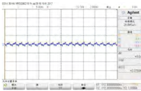
图7 57CM23电机在900rpm时的绕组电流波形
