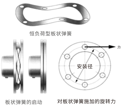
恒负荷板状弹簧工作原理图
