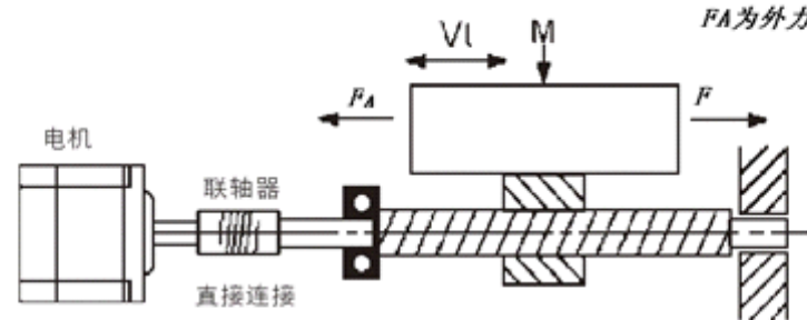
图1：丝杠水平运动
